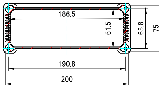
A-A ( 1 : 3.5 )
