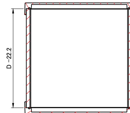
C-C ( 1 : 3.5 )
